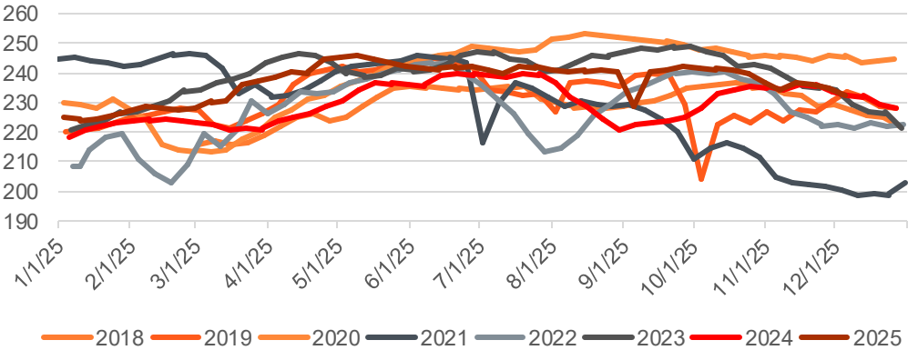
铁水产量
