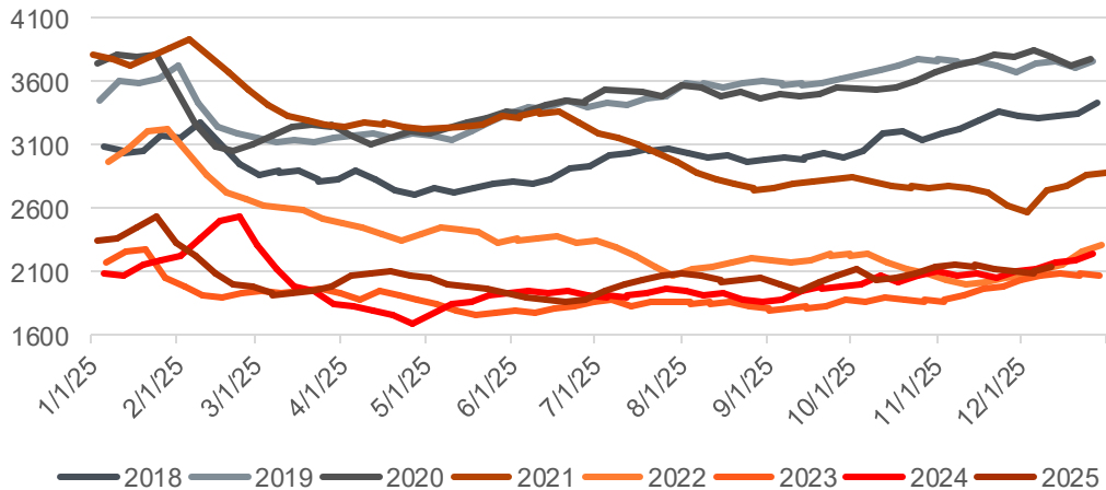
焦煤总库存
