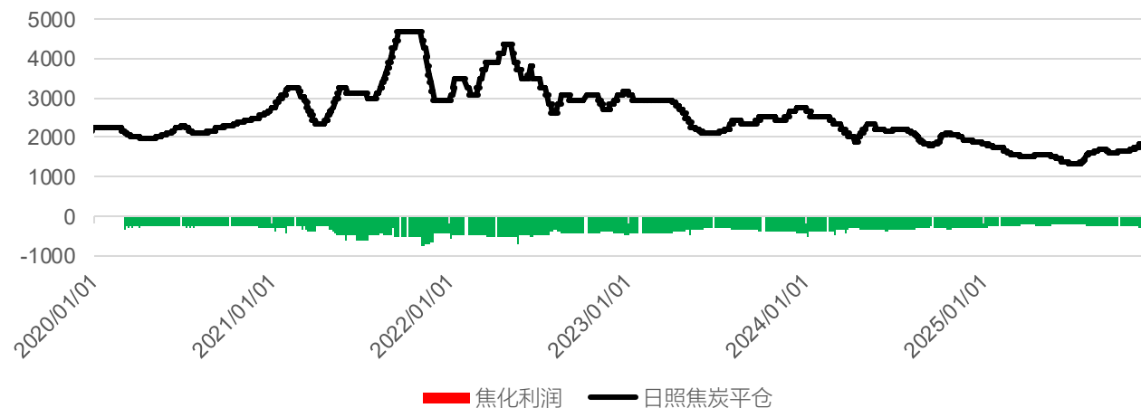
焦炭利润
