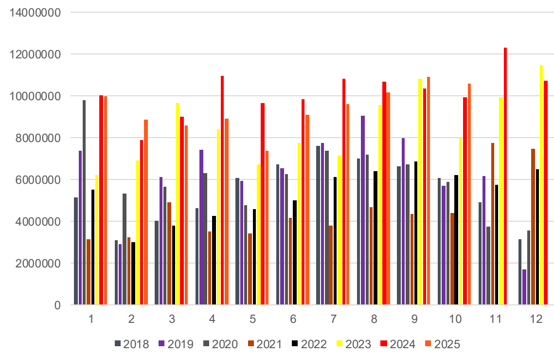
焦煤进口
