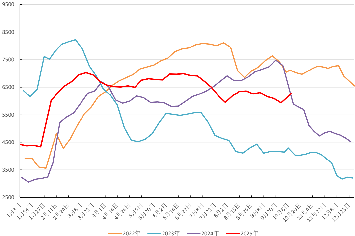
全国浮法玻璃生产企业库存
