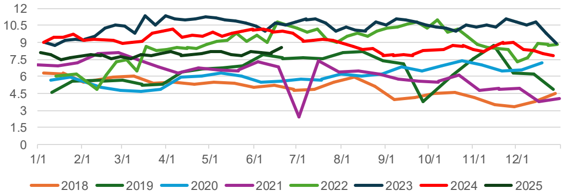
64家钢厂国产粉矿日耗（万吨）
