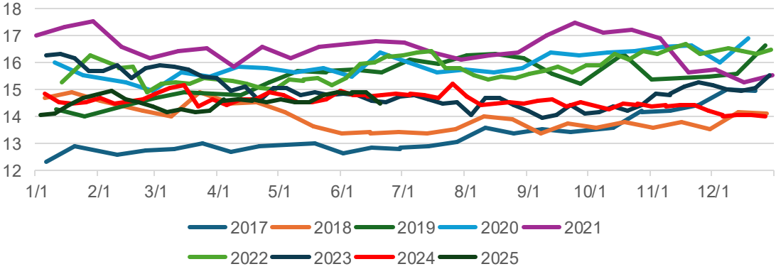
球团矿入炉配比 (%)
