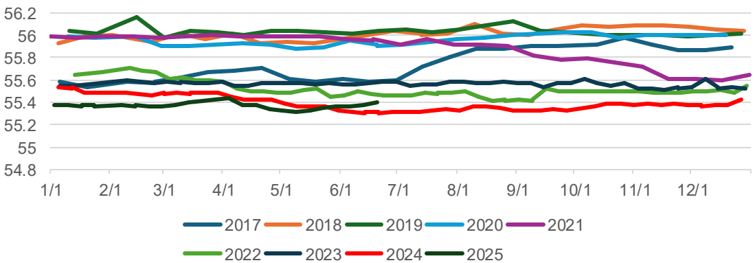
烧结矿入炉品位（%）
