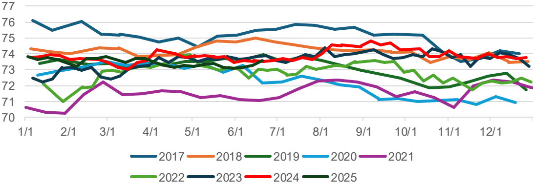
烧结矿入炉配比 (%)
