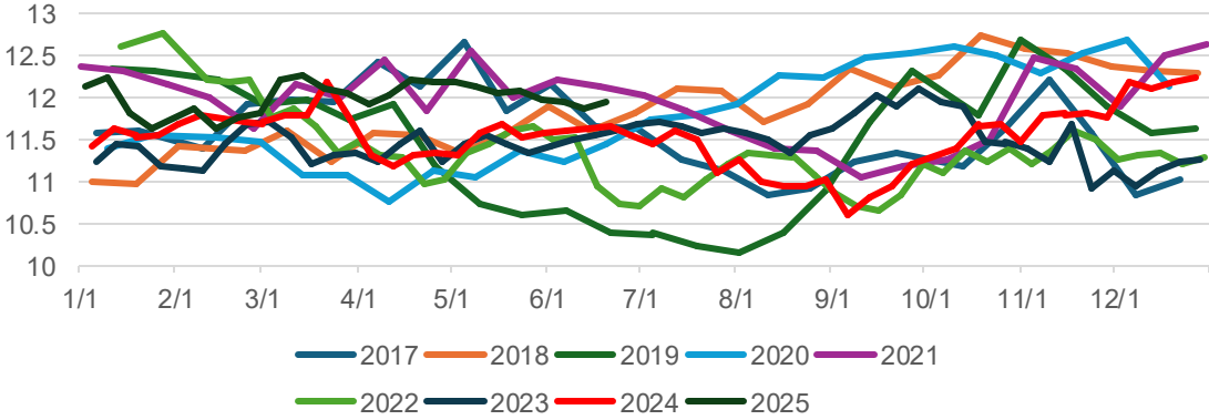
块矿入炉配比 (%)
