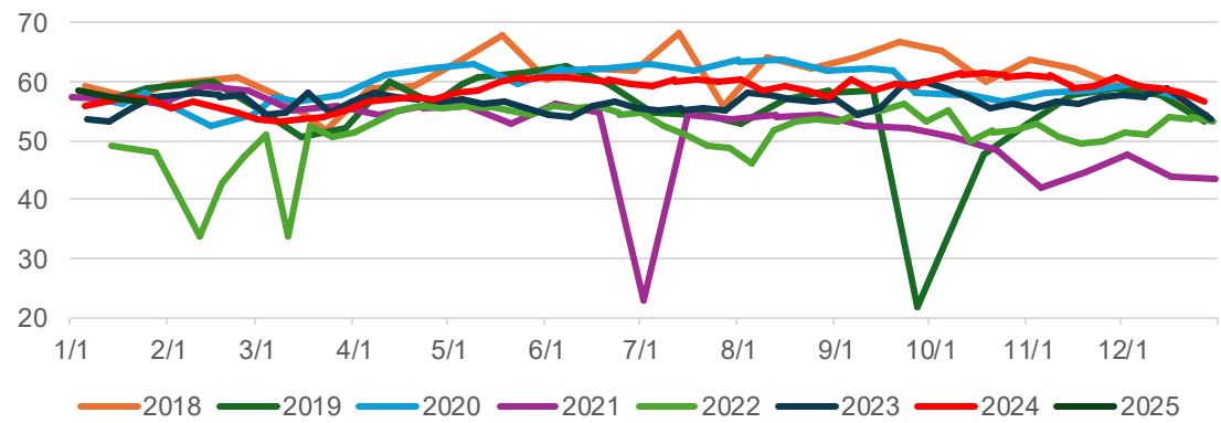
64家钢厂进口粉矿日耗（万吨）
