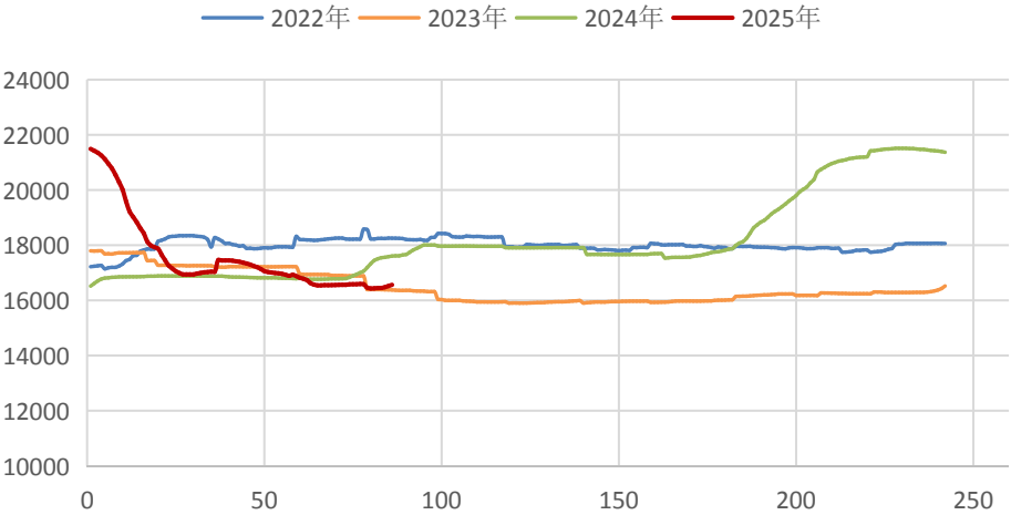
电解铝理论成本：元/吨
