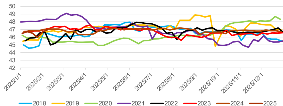
钢厂焦化日均产量
