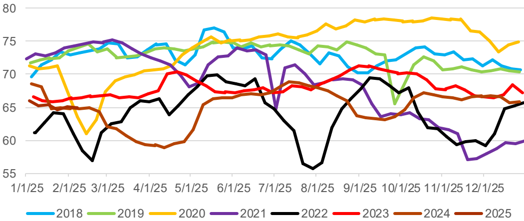
独立焦化厂焦炭日均产量
