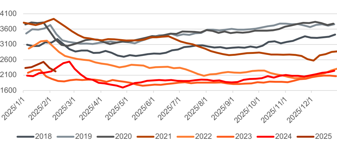
焦煤总库存
