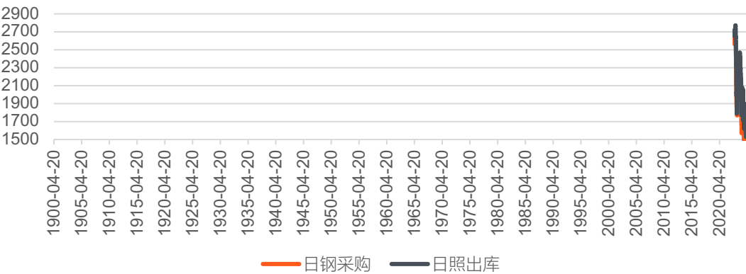
焦炭价格
