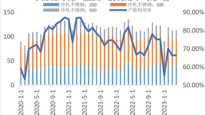
不锈钢冷轧产量及产能利用率 (万吨)
