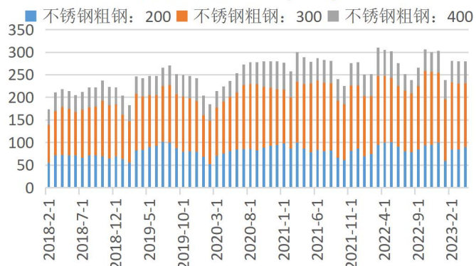
中国不锈钢产量 (万吨)
