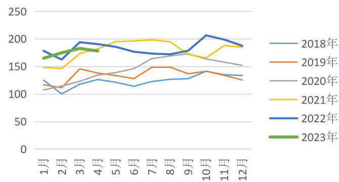
不锈钢300产量: 中国+印尼 (万吨)
