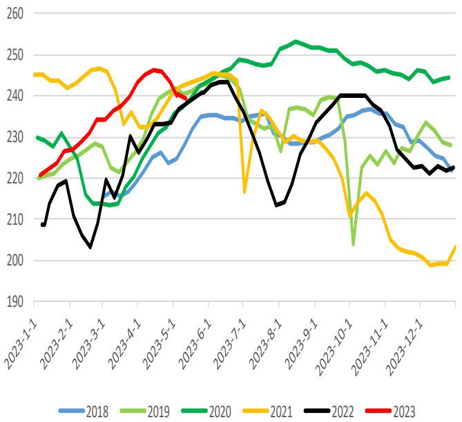
铁水产量
