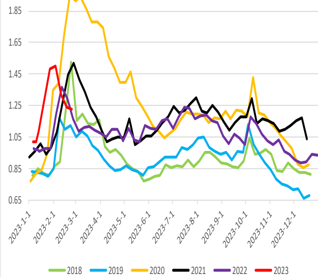
热卷库销比
