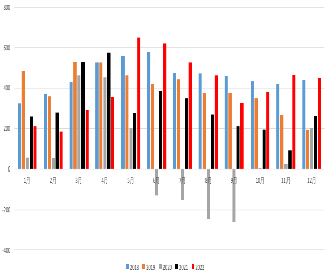
钢材净出口
