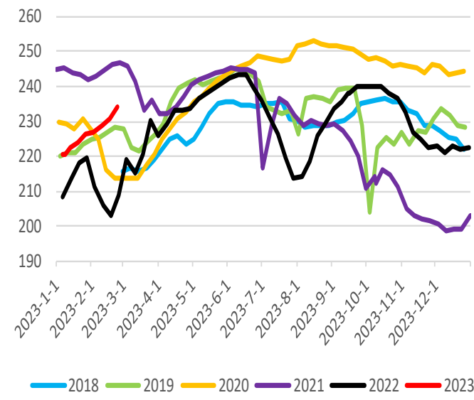
铁水产量
