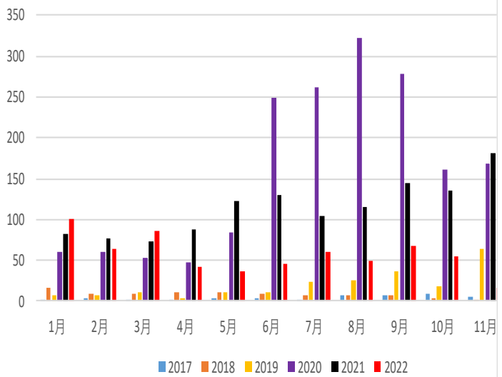
进口钢坯
