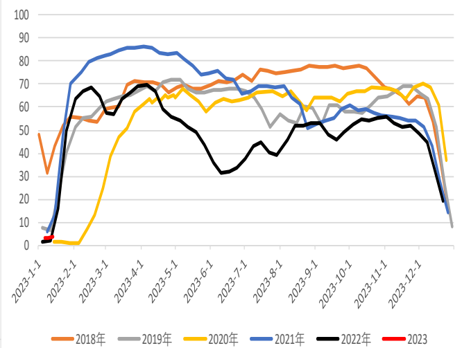
农历电弧炉产能利用率
