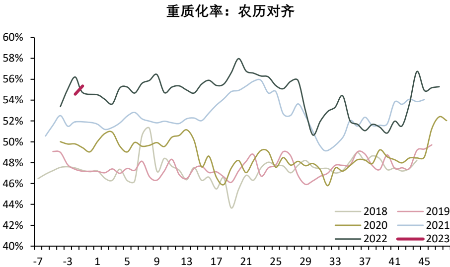
Figure 5 重质化率 (%)
