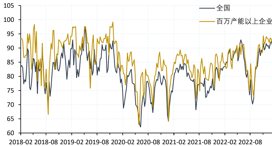
Figure 4 隆众开工率（%）
