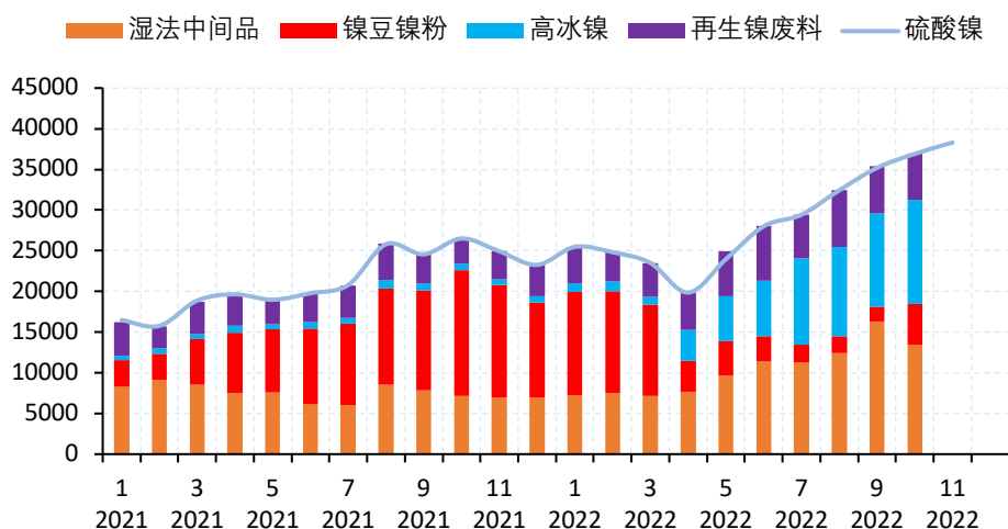
硫酸镍产量
