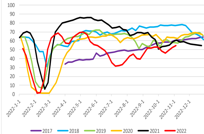
电弧炉产能利用率
