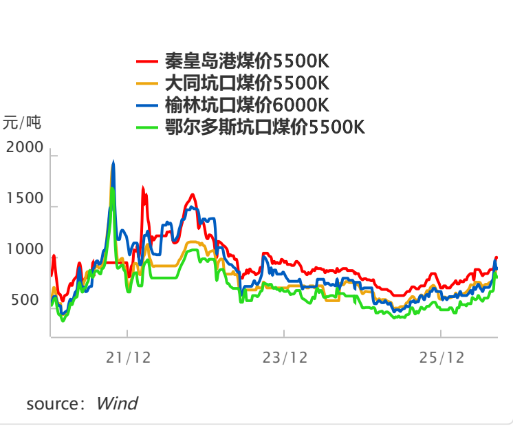
动力煤价格.
