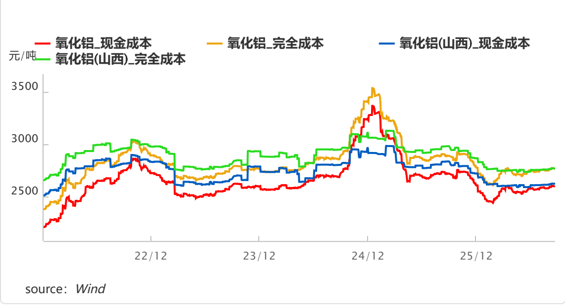
氧化铝成本.
