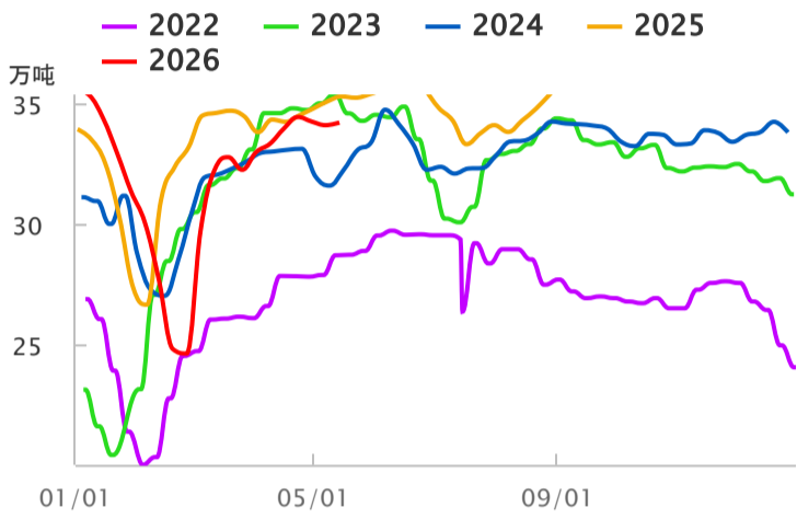
铝棒产量 (周) 季节性.
