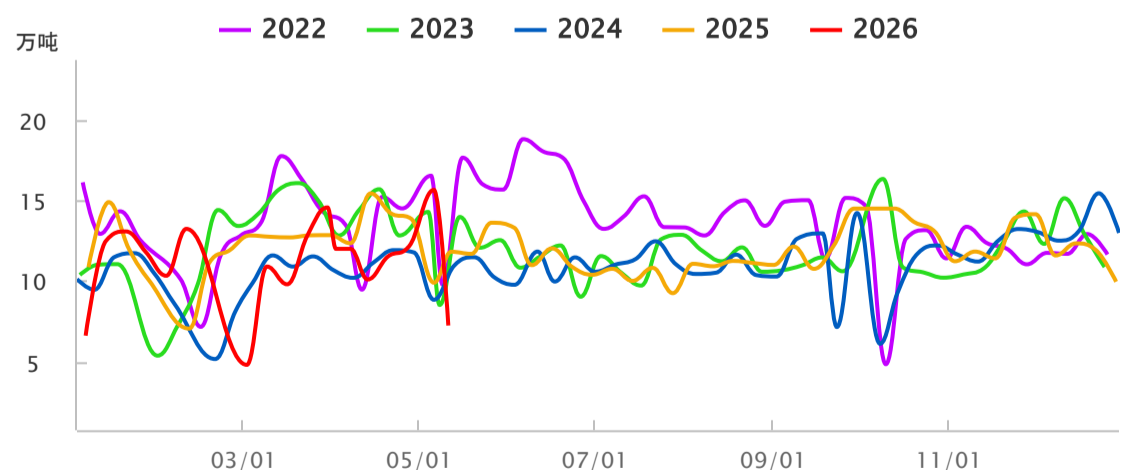
铝锭周度出库量季节性.
