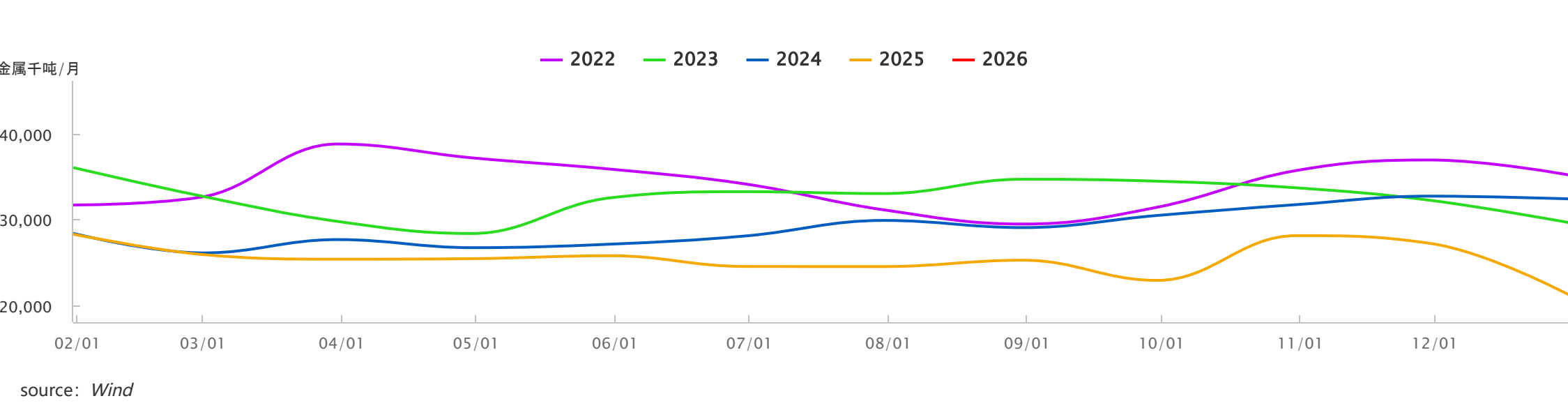
中国镍铁月度产量季节性.
