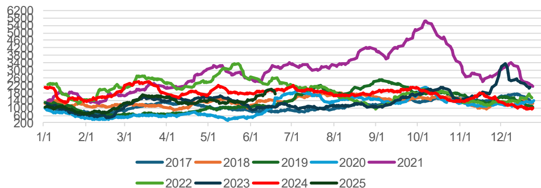
BDI指数
