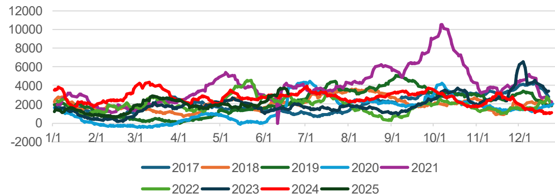
BCI指数
